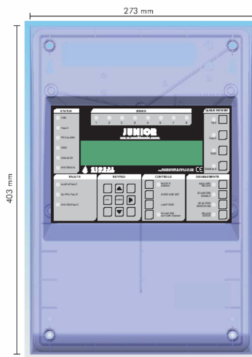
ELŐLNÉZET
