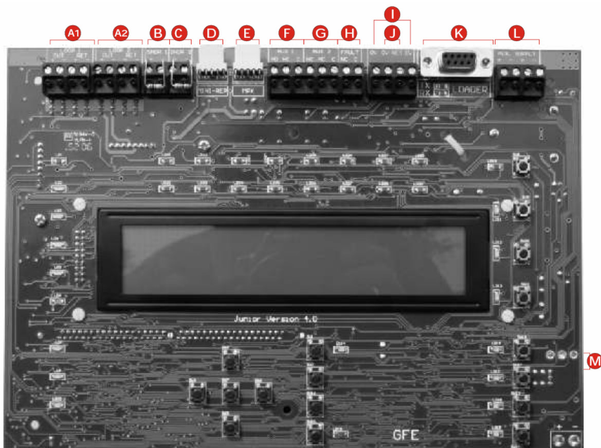
JUNIOR KÖZPONTI PANEL
