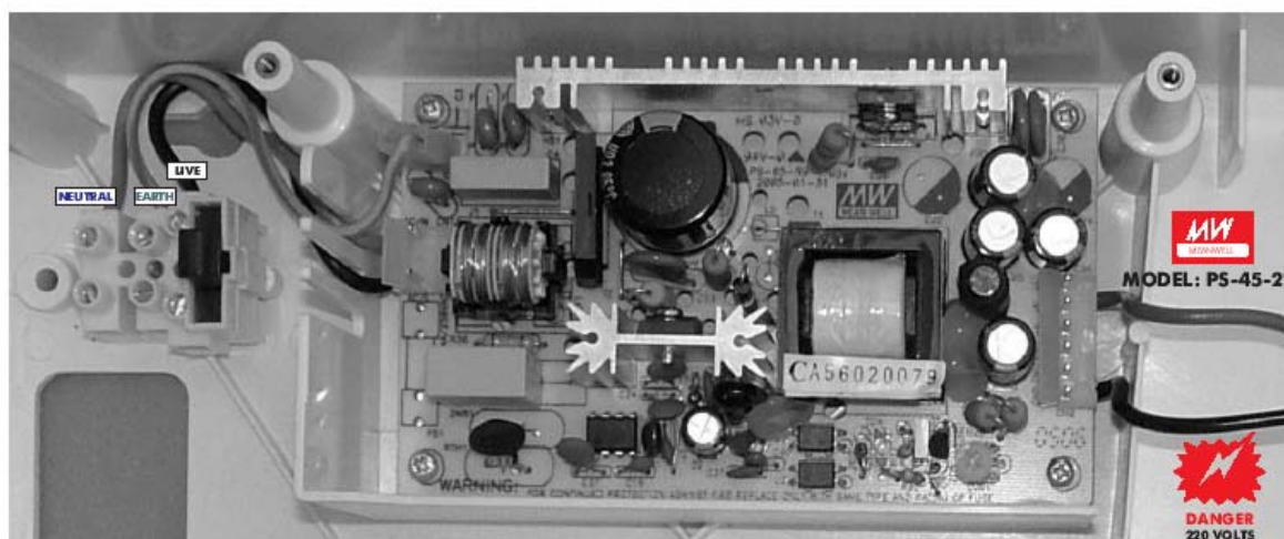
Tápellátás részletezése – MEANWELL Modell: PS-45-27
