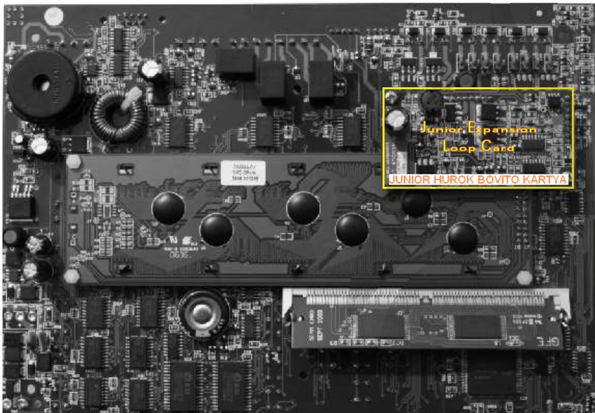
HÁTUL NÉZET
