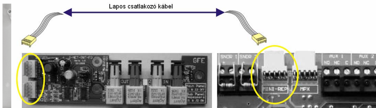
JUNIOR PANEL CSATLAKOZTATÁS
